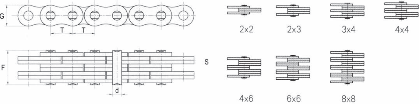
Serie LH (DS/ISO 4347 Amerikansk standard B29-8)
