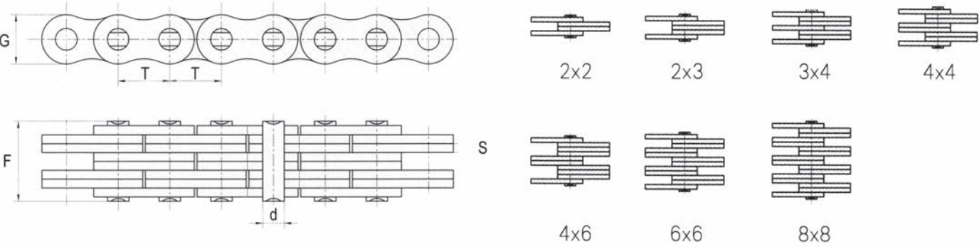
Serie LH (DS/ISO 4347 Amerikansk standard B29-8)
