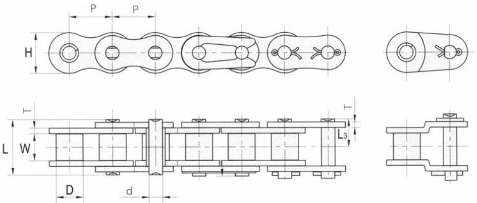
ISO 606 Type A / DIN 8188 / Amerikansk Standard B29-1
