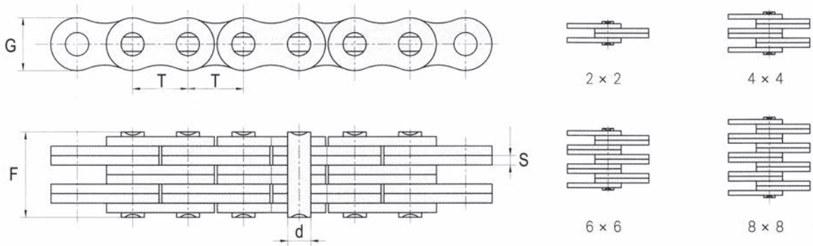
Serie LL (DS/ISO 4347)
